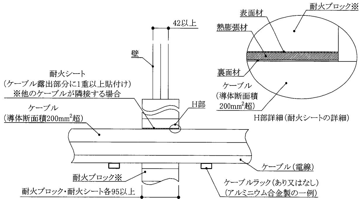
E-E断面図 (他のケーブルが隣接する場合におけるケーブル(導体断面積200mm 2 超)と耐火シートの施工例)
