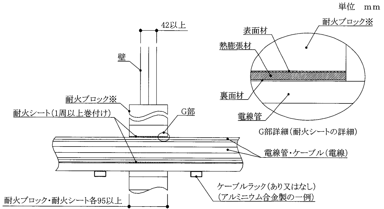
D-D断面図 (電線管への耐火シート1周巻きの施工例)
