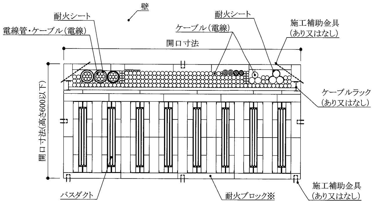
立面図(矩形の一例)
