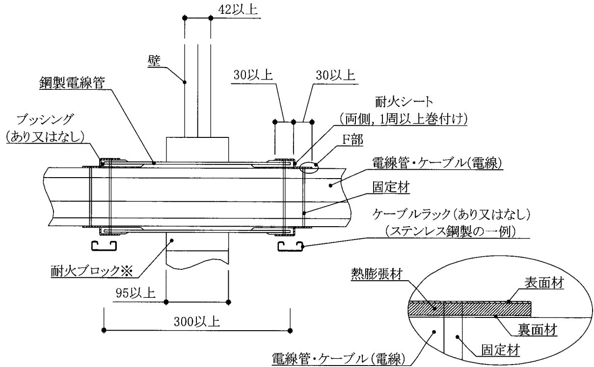
F部詳細(耐火シートの詳細)
