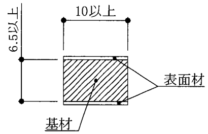
耐火マット用補助充填材断面図の一例
