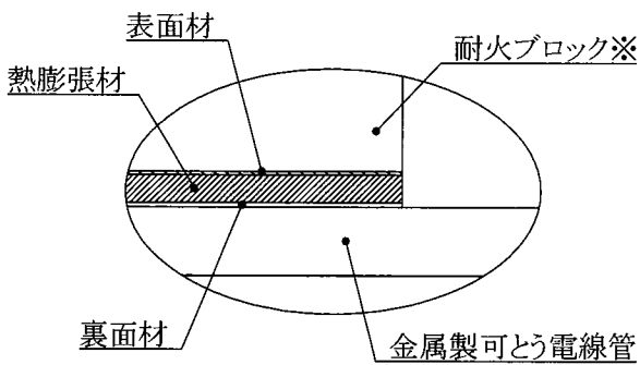
D部詳細(耐火シートの詳細)
