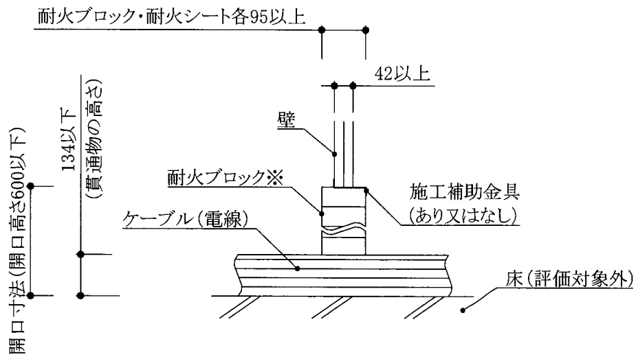
断面図(床置き工法の例)
