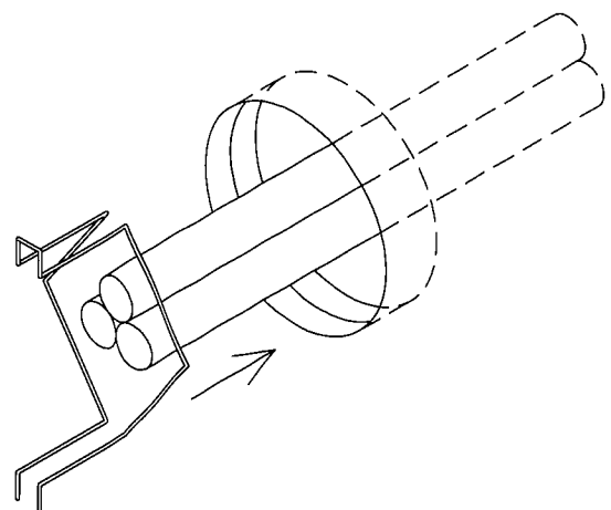
施工補助金具(円形開口用)の一例
