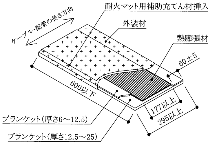
耐火マット詳細図の一例
